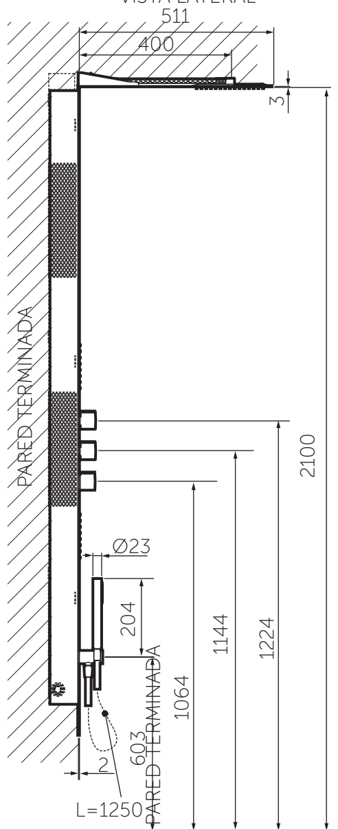
VISTA LATERAL
