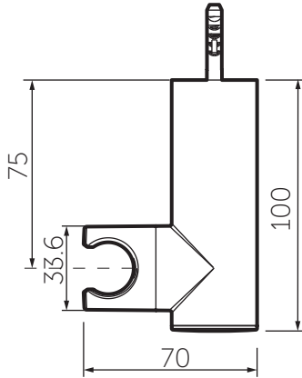
VISTA SUPERIOR
