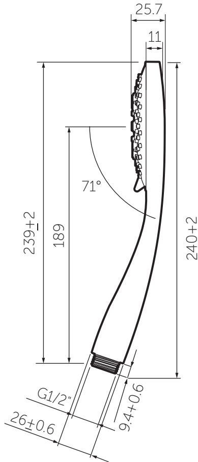
VISTA LATERAL
