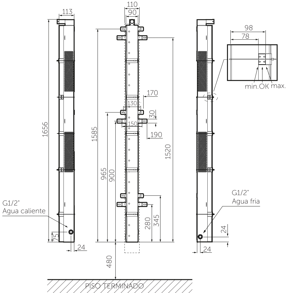
VISTA LATERAL
