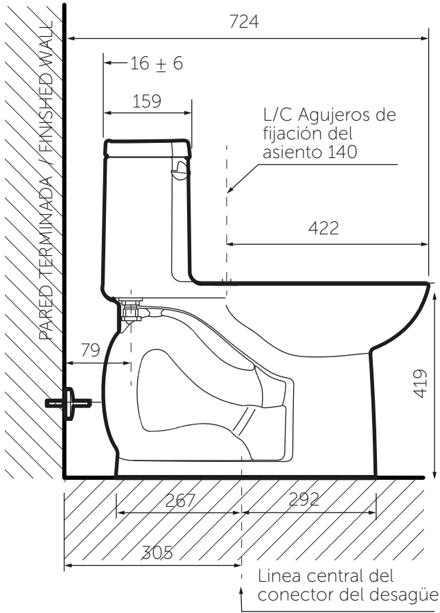
VISTA LATERAL
